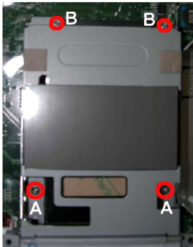
Fig. 29 HDD Holder
